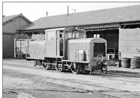
725 CF – ROMORANTIN (41) Locotracteur BA 14 au dépôt. Photo Jacques BAZIN (†) – 1963.
